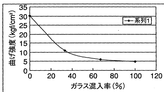
天然砂利+ガラス配合曲げ強度
